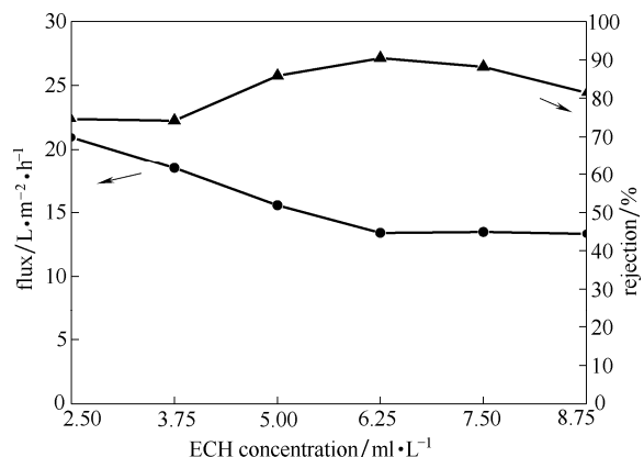
图 6 ECH 的用量对复合膜的截留率和渗透通量的影响
