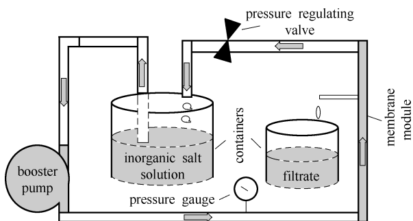
图 2 NF 膜评价系统示意图
