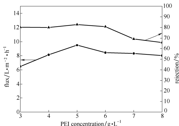
图 3 PEI 溶液的浓度对复合膜的截留率和渗透通量的影响
