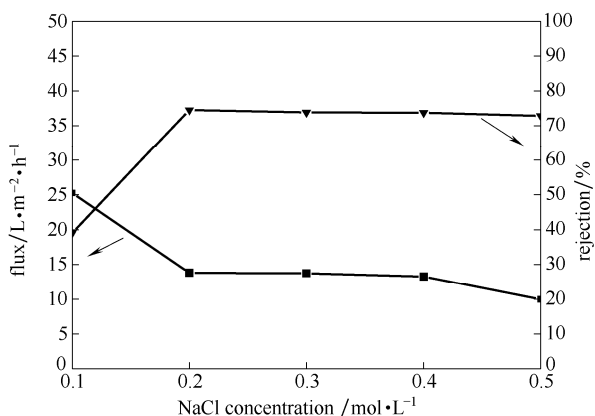
图 4 NaCl 的含量对复合膜的截留率和渗透通量的影响
