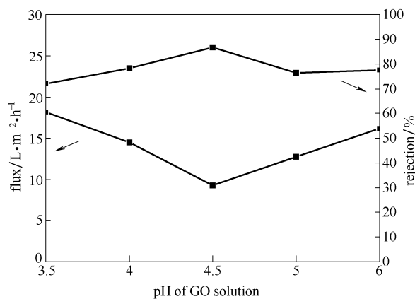
图 5 GO 溶液的 pH 对复合膜的截留率和渗透通量的影响
