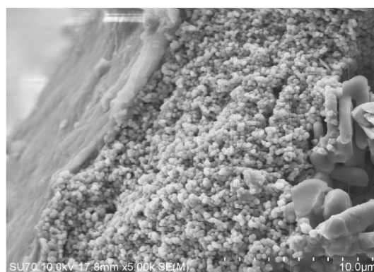
(d) cross-section image of composite NF membrane
