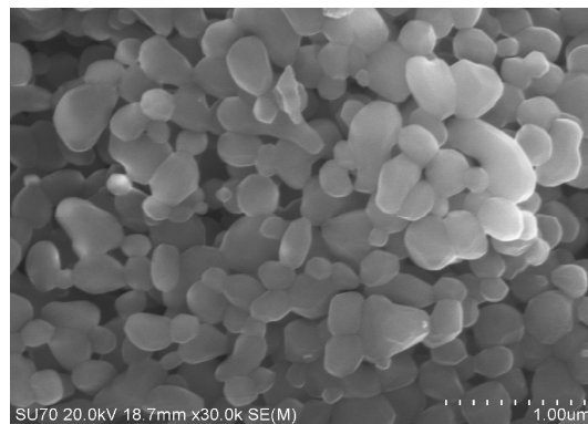
图 12 0.1 \mu\text{m} 多孔氧化铝基膜的形貌
